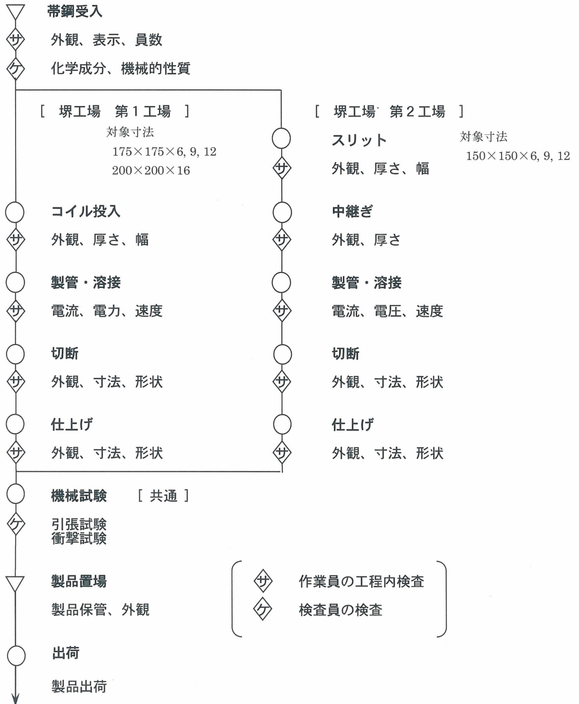
図 2 製造工程及び検査工程
